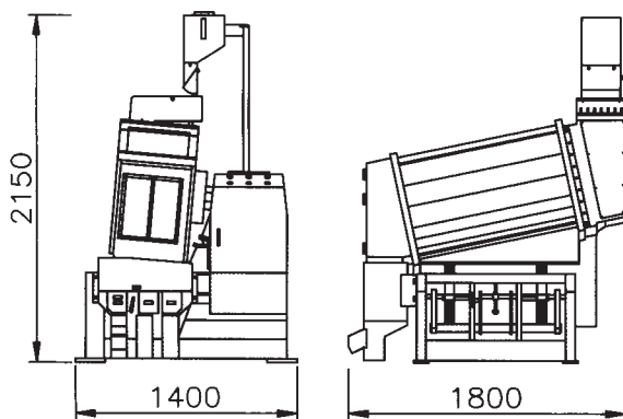
型號：PS-60
