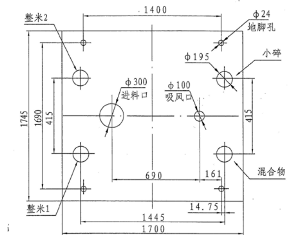
(外型尺寸與地腳安裝圖)
